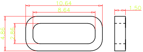
建议的胶圈尺寸
